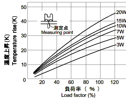
温度上昇 (参考)MQS,MQR Temperature rise (ref.)MQS,MQR
